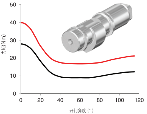
ITS900(4号力)力矩图
