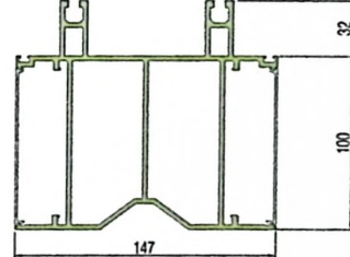
幕墙横梁•M140227 \delta=2.5 5.298 \frac{kg}{m} 横梁扣盖•Y140-286 \delta=1.2 0.322 \frac{kg}{m}
