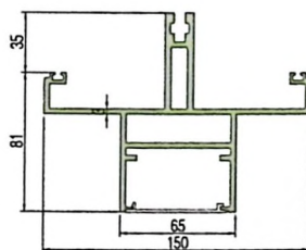
幕墙横梁•M125-11 \delta=3.0 4.440 \frac{kg}{m} 横梁扣盖•Y110-08 \delta=1.5 0.270 \frac{kg}{m}
