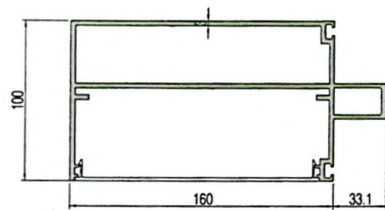
幕墙横梁•M140192 \delta=2.5 3.784 \frac{kg}{m} 横梁扣盖•Y150204 \delta=1.3 0.240 \frac{kg}{m}
