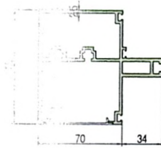
幕墙横梁•JXMQ16007 \delta=3.0 5.035 \frac{kg}{m} 横梁扣盖•JXMQ16008 \delta=2.0 0.865 \frac{kg}{m}
