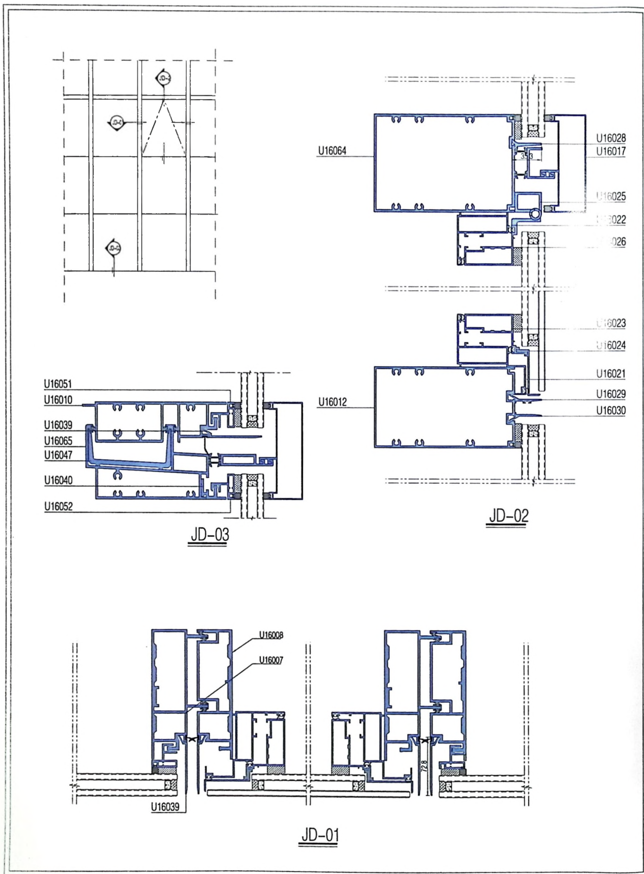
160单元式幕墙结构图一
