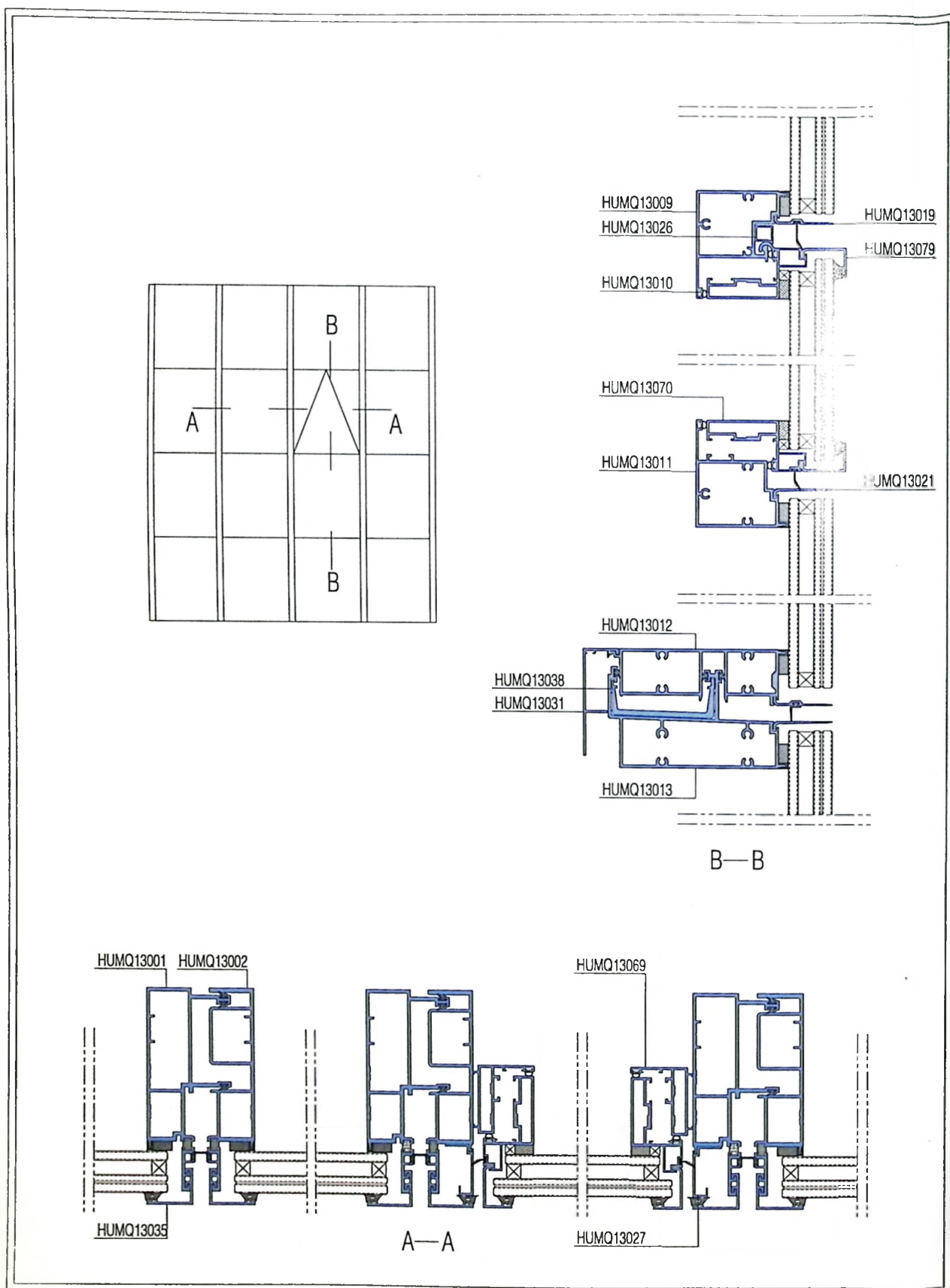
130单元式幕墙结构图
