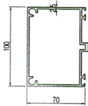
幕墙横梁•M160-148 \delta=2.5 3.303 \frac{kg}{m} 横梁扣盖•M160-15 \delta=1.2 0.218 \frac{kg}{m}
