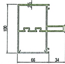
幕墙横梁•NTMQ20002 \delta=4.5 4.815 \frac{kg}{m} 横梁扣盖•NTMQ20003 \delta=1.2 0.256 \frac{kg}{m}
