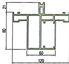
幕墙横梁•M125-11 \delta=3.0 4.440 \frac{kg}{m} 横梁扣盖•Y110-08 \delta=1.5 0.270 \frac{kg}{m}
