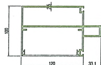
幕墙横梁•JXMQ16029 \delta=2.5 3.793 \frac{kg}{m} 横梁扣盖•JXMQ16030 \delta=2.0 0.649 \frac{kg}{m}
