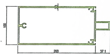
幕墙横梁•M140227 \delta=2.5 5.298 \frac{kg}{m} 横梁扣盖•Y140-286 \delta=1.2 0.322 \frac{kg}{m}
