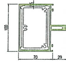
幕墙横梁•JXMQ16029 \delta=2.5 3.793 \frac{kg}{m} 横梁扣盖•JXMQ16030 \delta=2.0 0.649 \frac{kg}{m}
