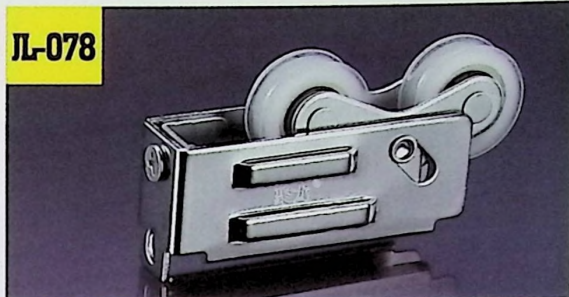
名称: 聚龙21号双轮 Size: 26.0X19.0X22.0mm
