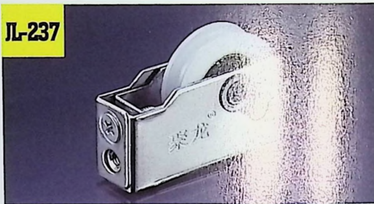
名称: 聚龙阳江70单轮 Size: 25.3X13.7X15.5mm
