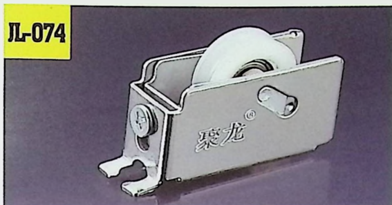
名称: 聚龙18号单轮 Size: 27.0X18.0mm
