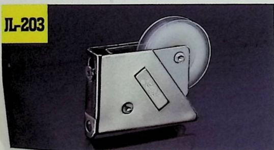
名称: 聚龙88系列单轮 Size: 37.5X13.3X15.0mm
