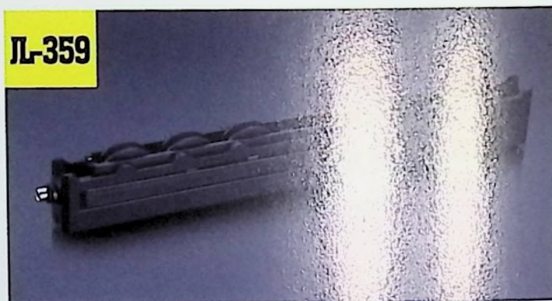
名称:出口21号六轮 Size:33.5X21.8X22.5mm
