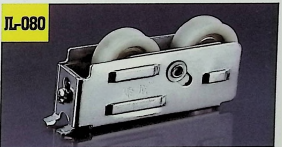
名称: 聚龙23号双轮 Size: 32.0X21.5X24.5mm
