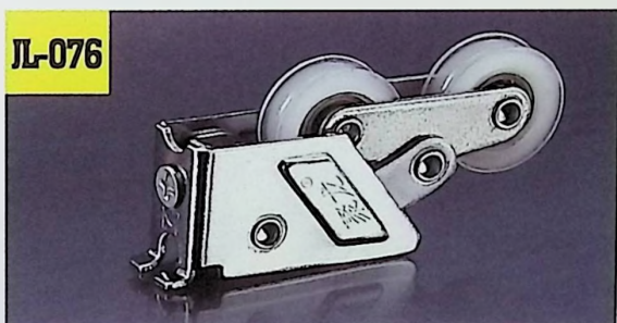
名称: 聚龙19号双轮 Size: 26.0X17.5X19.5mm
