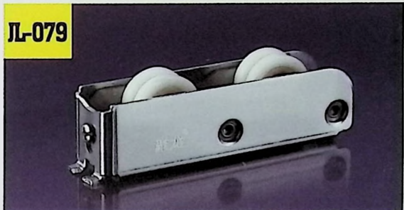
名称: 聚龙22号双轮 Size: 32.0x26.8mm
