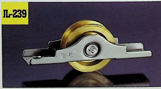
名称: 聚龙小一百单轮 Size: 15.8X13.5X14.5mm
