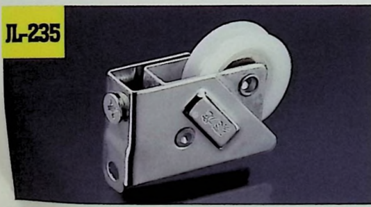
名称: 聚龙活动828单轮 Size: 27.0X13.5X14.5mm
