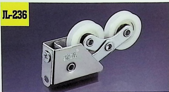
名称: 聚龙活动828双轮 Size: 27.0X14.5mm
