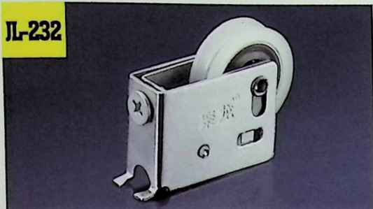
名称: 聚龙828单轮有孔开叉 Size: 27.5X13.5X14.5mm
