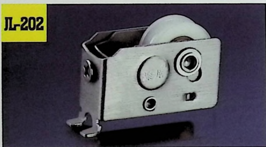
名称: 聚龙凤铝888单轮开叉 Size: 25.2X17.5X19.8mm
