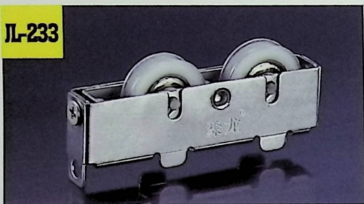
名称: 聚龙旧828双轮 Size: 26.8X14.5mm
