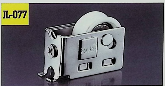
名称: 聚龙20号单轮 Size: 26.0X18.3X20.3mm
