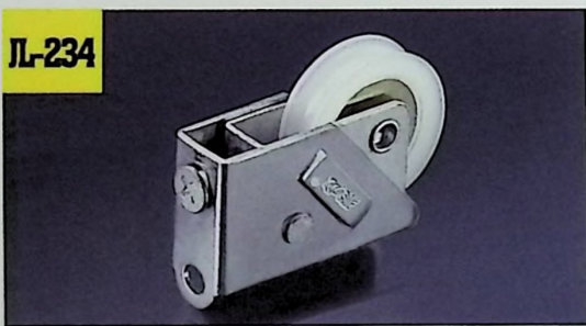
名称: 聚龙活动818单轮 Size: 25.0X13.0X14.5mm
