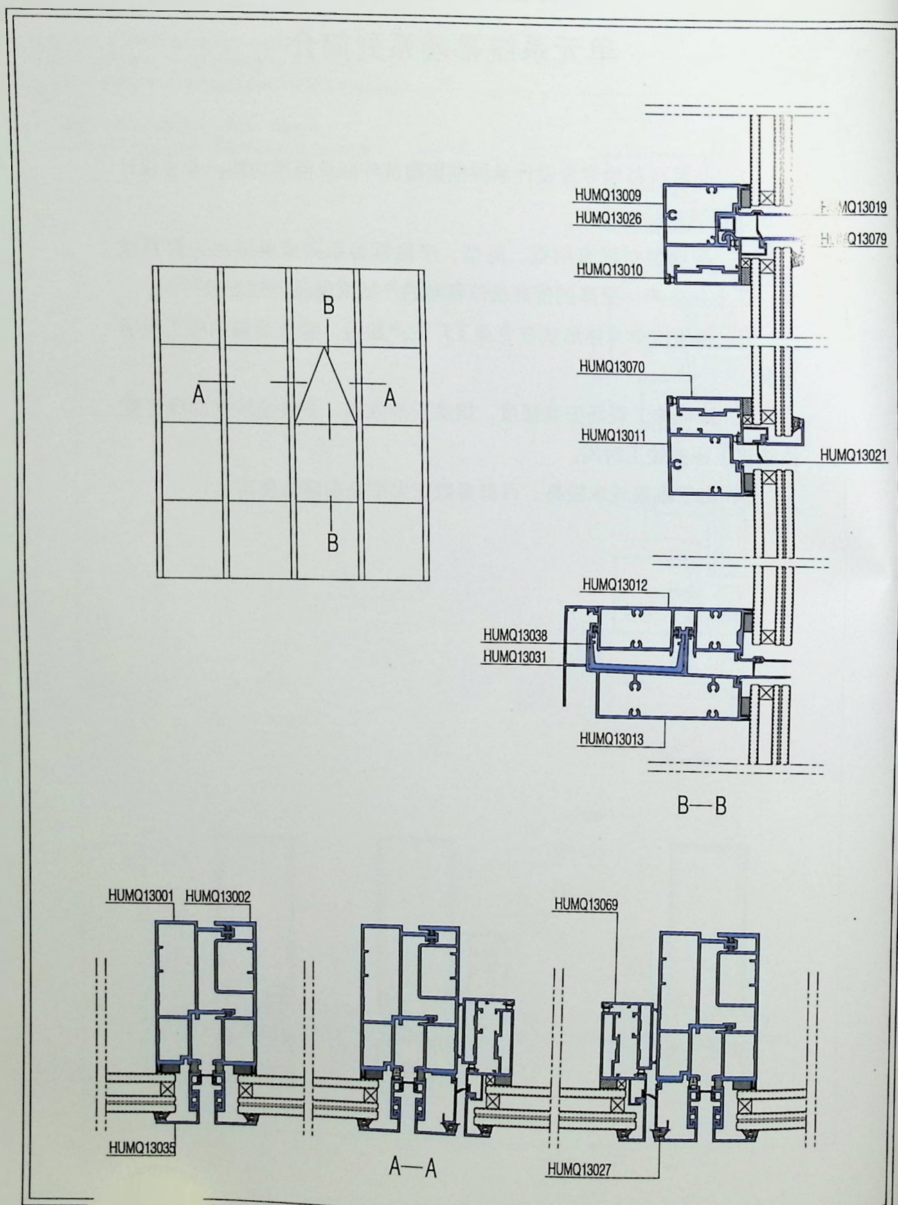
130单元式幕墙结构图
