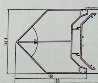
转角扣盖•M18093 \delta=2.5 4.087 \text{kg/m} 转角压板•M18094 \delta=4.0 2.041 \text{kg/m}
