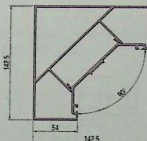
转角扣盖•JXMQ17023 \delta=2.2 3.531 \text{kg/m} 转角压板•JXMQ17024 \delta=2.5 1.283 \text{kg/m}
