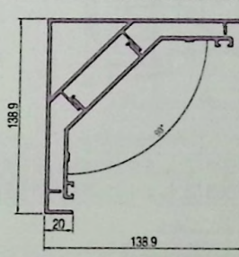
转角扣盖•JXMQ17023 \delta=2.2 3.531 \text{kg/m} 转角压板•JXMQ17024 \delta=2.5 1.283 \text{kg/m}
