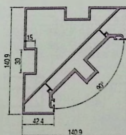
转角扣盖•M18093 \delta=2.5 4.087 \text{kg/m} 转角压板•M18094 \delta=4.0 2.041 \text{kg/m}
