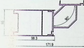
转角压板•TMQ022 \delta=3.0 2.269 \text{kg/m} 转角扣盖•TMQ021 \delta=1.5 1.360 \text{kg/m}
