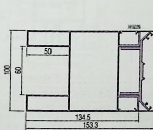
转角扣盖•H16025 \delta=1.4 2.909 \text{kg/m} 转角压板•H16027 \delta=3.0 1.317 \text{kg/m}
