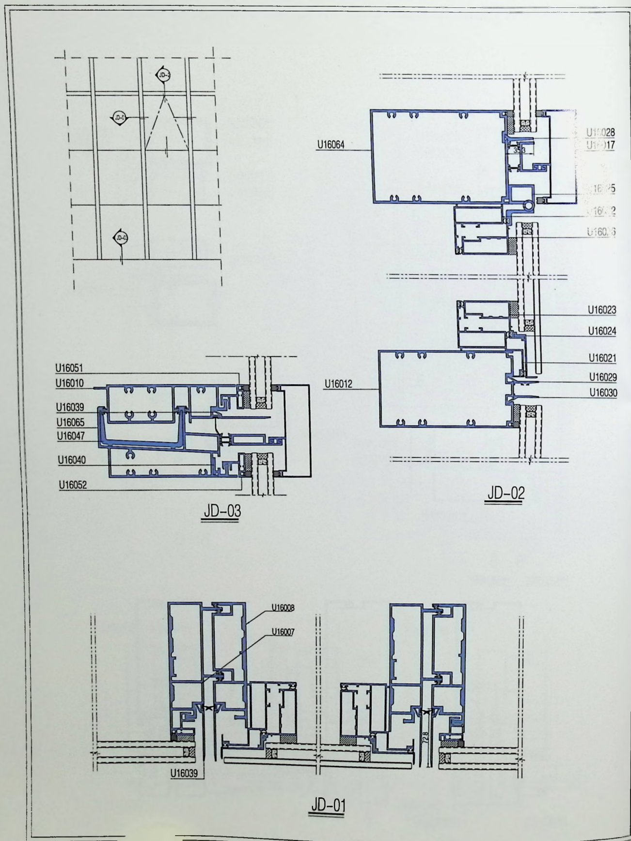
160单元式幕墙结构图一
