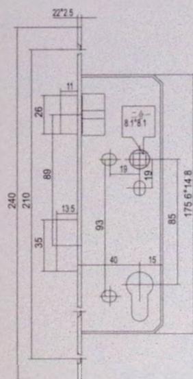
8540 双活双快
