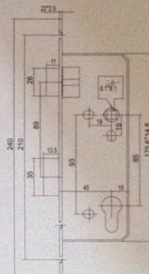
8545 双活双快
