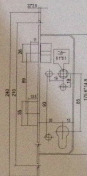
8535 双活双快
