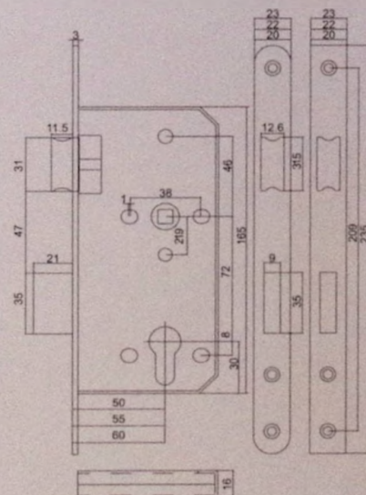
7255 快开
