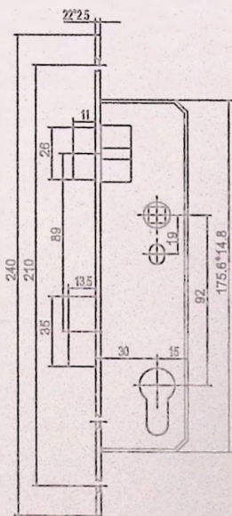
9230 单点
