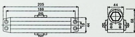
CY-063 三角型闭门器 Triangle door closer
