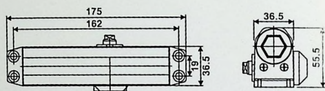
CY-165F 方形闭门器 (B3) Hexagonal door closer (B3)
