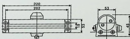
CY-080 圆型隐藏闭门器 Concealed overhead door closer
