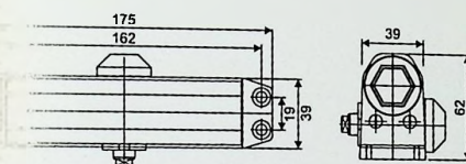
CY-165FBC 方形闭门器 (B3) Hexagonal door closer (B3)
