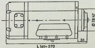
平面图 HSK 32E / HSK 40E
