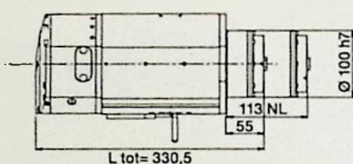
平面图 PX NC/NL
