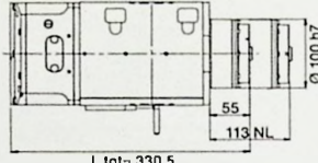
平面图 HX NC/NL
