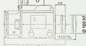
平面图 HX 3C NC/NL
