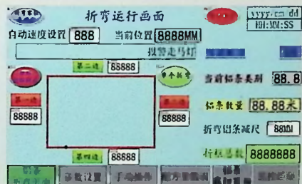
人机界面
