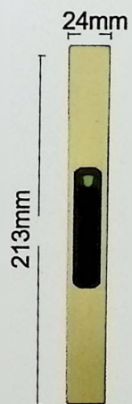
JG205 小方锁 (拉丝金/ 拉丝银 / 枪黑)
